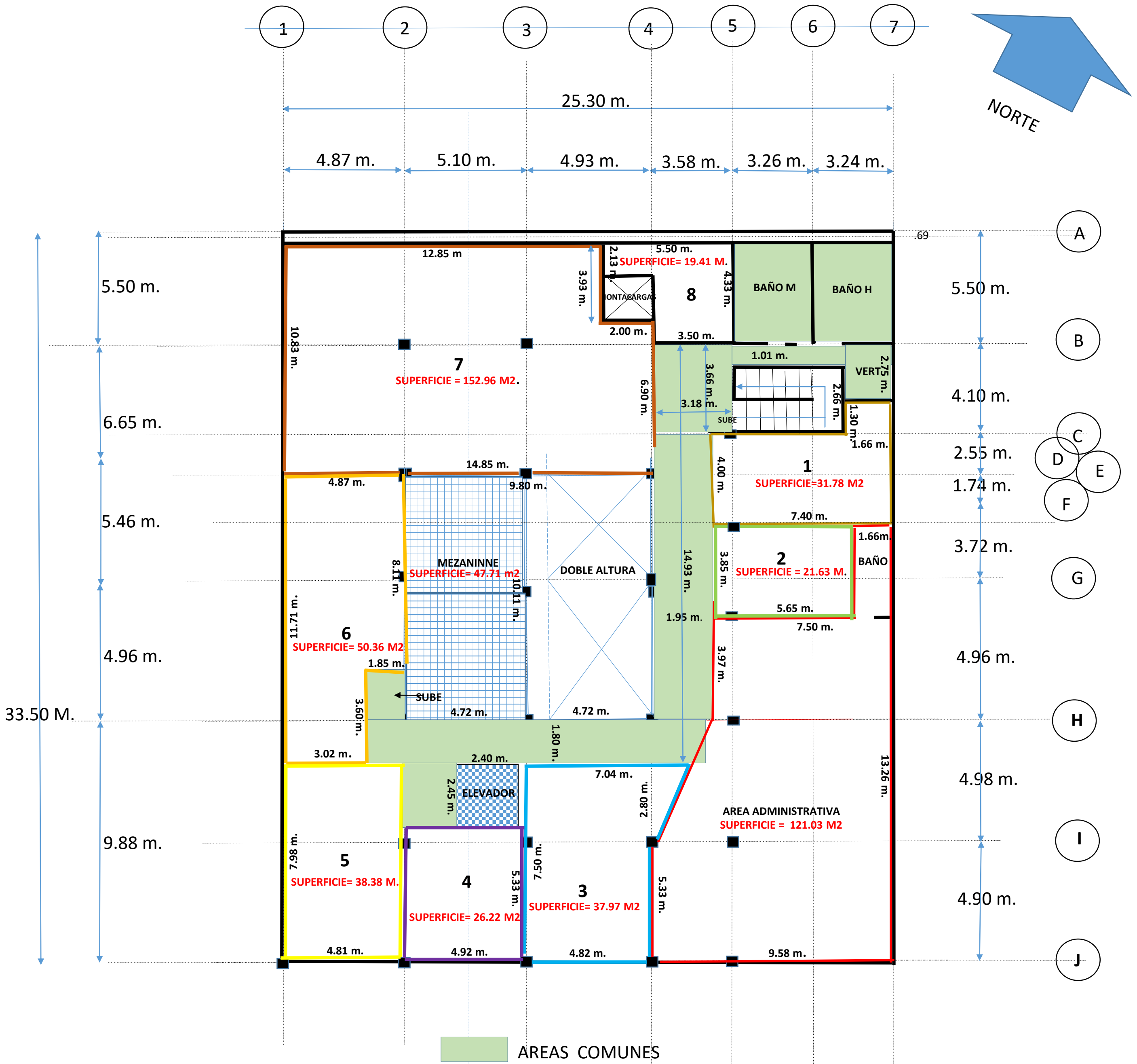
PLANTA ARQUITECTONICA TERCER PISO
